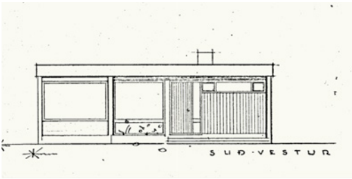
Hvoll, úr ódagsettum aðaluppdrætti
