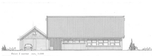
Blikastígur 3, úr aðaluppdrætti frá 1982
