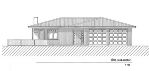
Fálkastígur 2, úr aðaluppdrætti frá 2002
