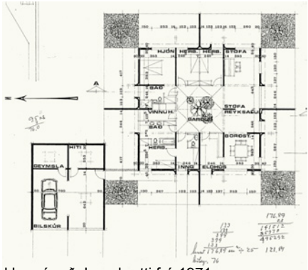
Stekkur, úr aðaluppdrætti frá 1971
