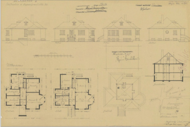
Hlyngerði 6 frá árinu 1945 eftir Einar Sveinsson arkitekt. Teikningavefur Reykjavíkurborgar.
