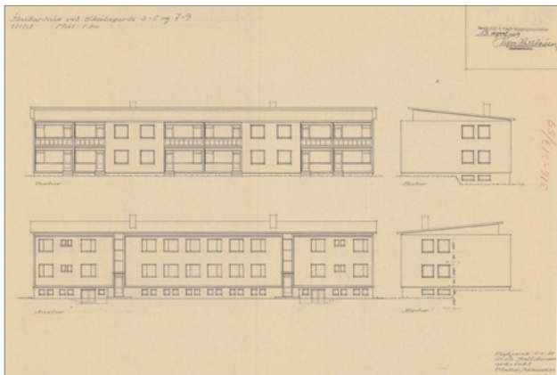
Teikningar Gísla Halldórssonar arkitekts og Ólafs Júlíussonar byggingafræðings af Skálagerði 3-5 og 7-9 frá árinu 1959. Teikningavefur Reykjavíkurborgar.
