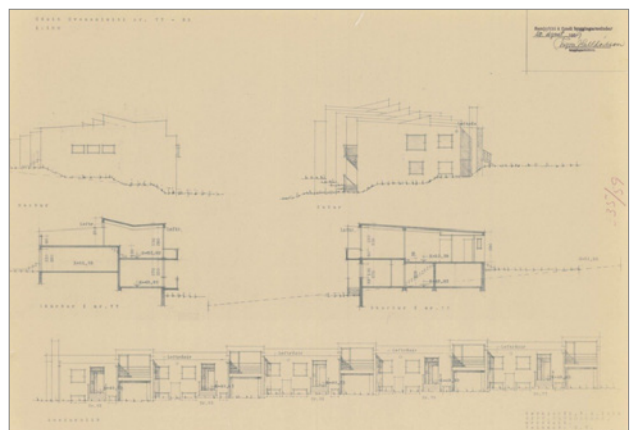
Teikningar að Hvassaleiti 77-85 frá árinu 1959 eftir Sigvalda Thordarson arkitekt. Teikningavefur Reykjavíkurborgar.
