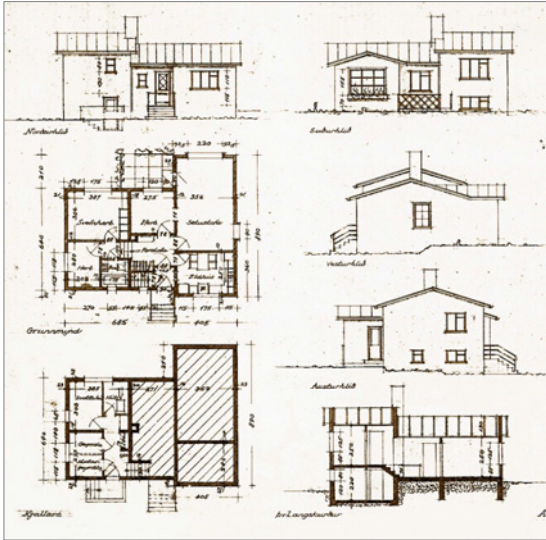
Heiðargerði 32. Teikning eftir Bárð Ísleifsson arkitekt frá árinu 1952. Teikningavefur Reykjavíkurborgar.
