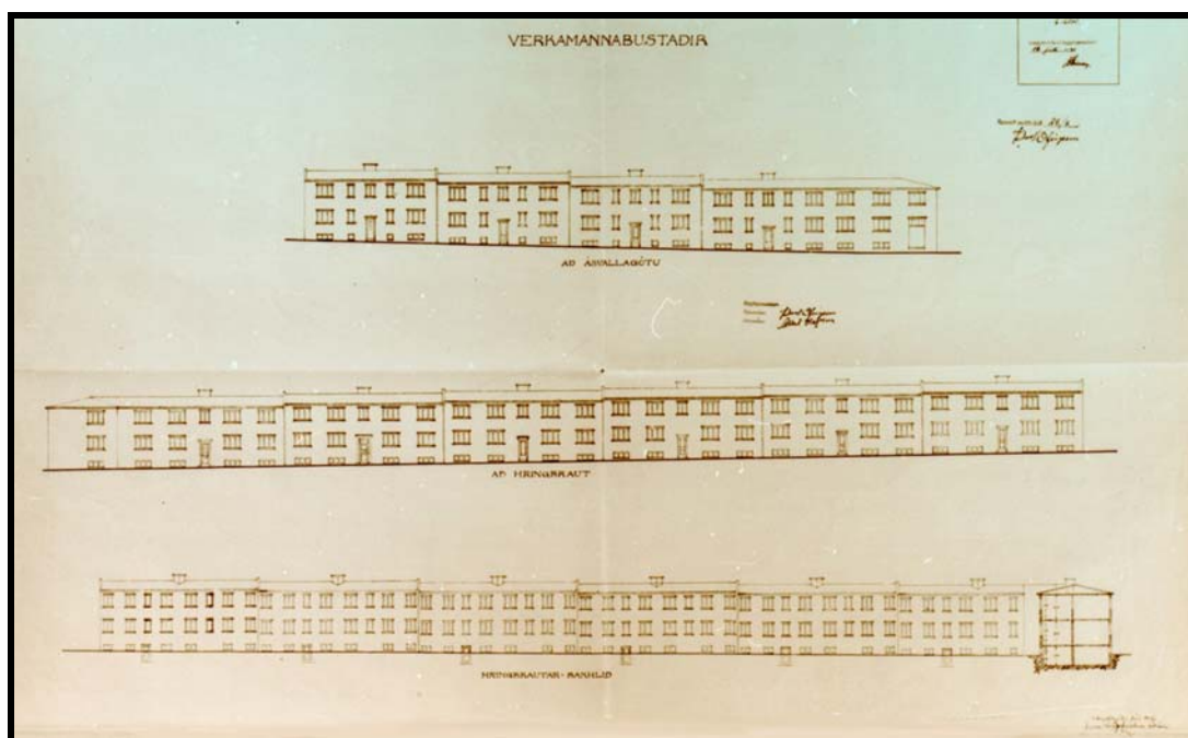
Ein af teikningum Einars Erlendssonar að fyrsta áfanga verkamannabústaðanna. 26
