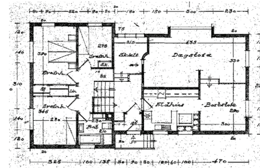
Mynd 37: Holtagerði 1. Grunnmyndir og ásýndir.
