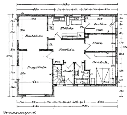
Mynd 36: Holtagerði 6. Grunnmyndir og ásýndir.
