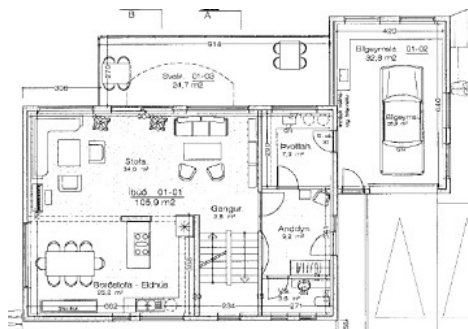
Grunnmynd jarðhæðar. Samp. 4.12.2012
