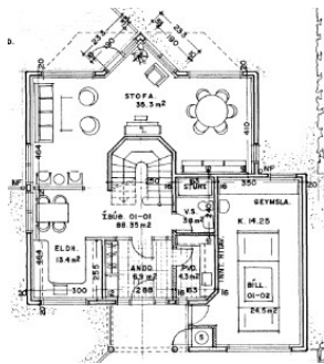
Grunnmynd 1. hæð. Samþykkt 12.11.2002
