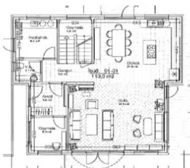
Grunnmynd 1. hæð. Samþykkt 9.2.2011
