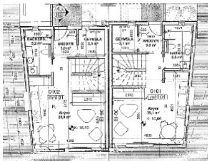
Grunnmynd 1. hæð
