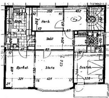
Teikning 2. og 3. hæð 2004
