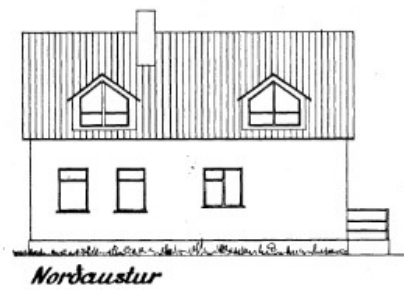
Teikning 1954
