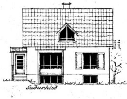
Teikning 1953
