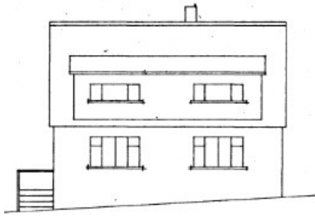
Teikning 1972
