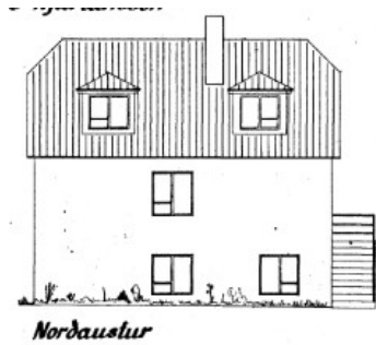
Teikning 1954
