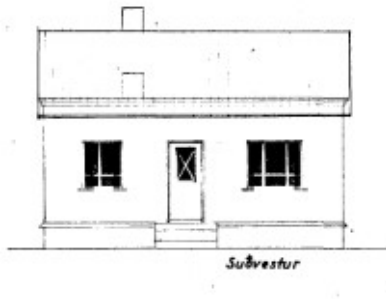
Teikning 1953
