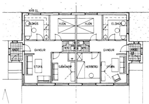
Grunnmynd teiknuð 1992
