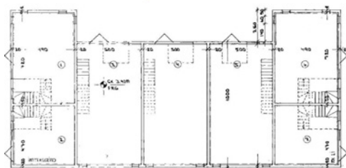
Grunnmynd, byggingarnefndarteikning
