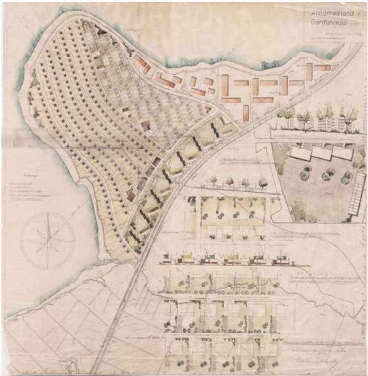
Arnarnesland í Garðahreppi Tillaga að skipulagi eftir Aðalstein Richer arkitekt (1958)
