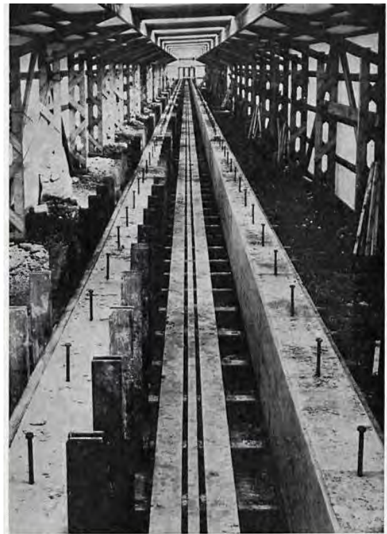
Framleiðsla á strengjasteypubitum á 75 m löngum spennibekk (Byggingariðjan hf.).
